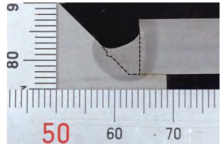
溶接部マクロ写真
