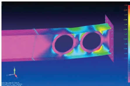
FEM解析の一例
