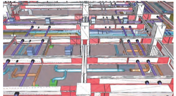
3Dモデルを設備CADに取り込みスリーブ配置を検討
