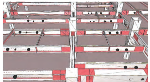
設備CADで検討後、出力されたスリーブ配置データをKAPに取り込みモデリング
